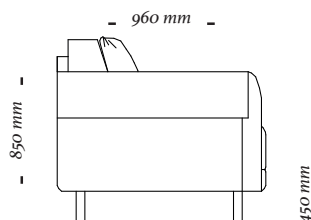
2 Lugares c/ 1 br 1320x960x850mm
