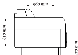
Poltrona c/ 1 br 1120x960x850mm
