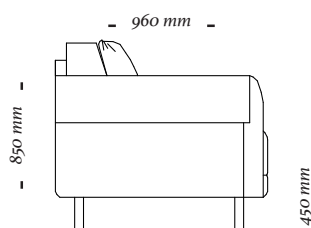
3 Lugares c/ 2 br 2640x960x850mm
