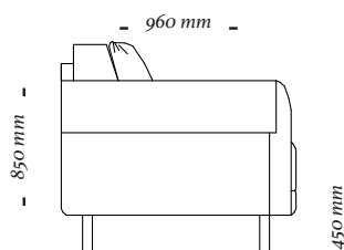
2 Lugares c/ 2 br 2240x960x850mm
